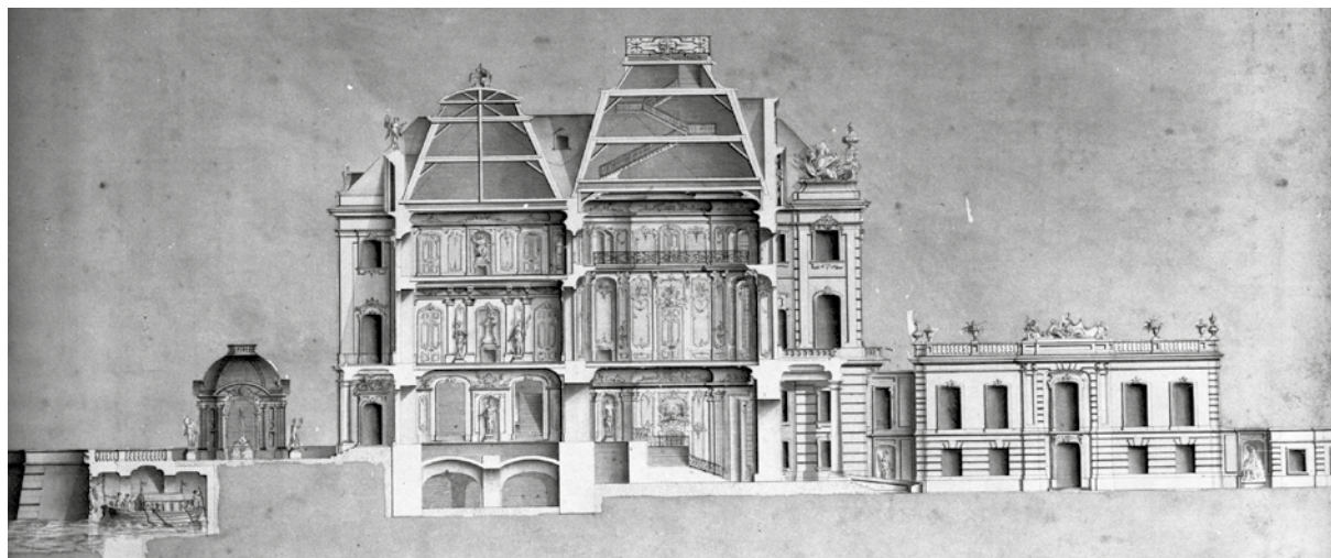
Az új kastély metszetábrázolása
