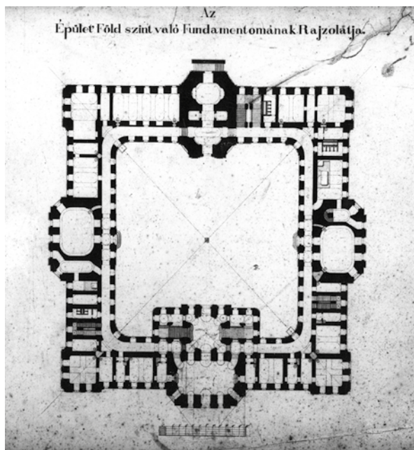
A líceum alaprajzi ábrázolása 1878-ból
