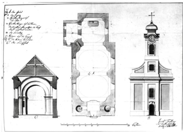
A nagyeztergári plébániatemplom Fellner által szignózott terve
