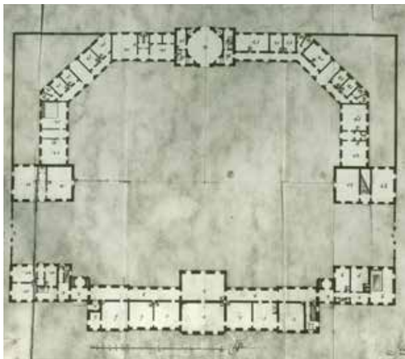
A tallósi Esterházy-kastély Fellner Jakab által aláírt alaprajza, átalakítási terve
