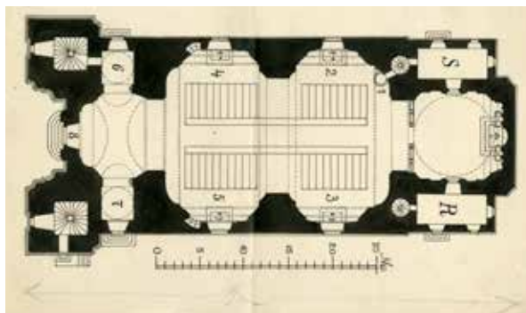
A tatai Szent Kereszt plébániatemplom alaprajza, Dornyay Béla rajzán
