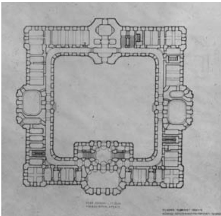
A Líceum épületének földszinti alaprajza (KDM REH)
