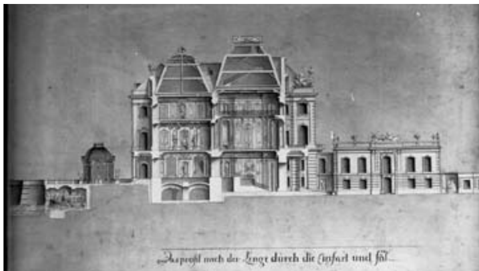
Fellner Jakob IV. tervvariáns a tatai várkastélyhoz. 1762–1763. É–D irányú keresztmetszet (KDM REH 2646–1218)
